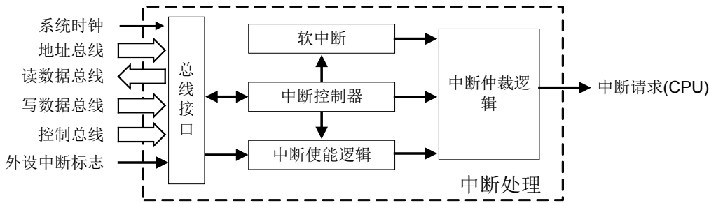
图 6-9 中断控制逻辑
