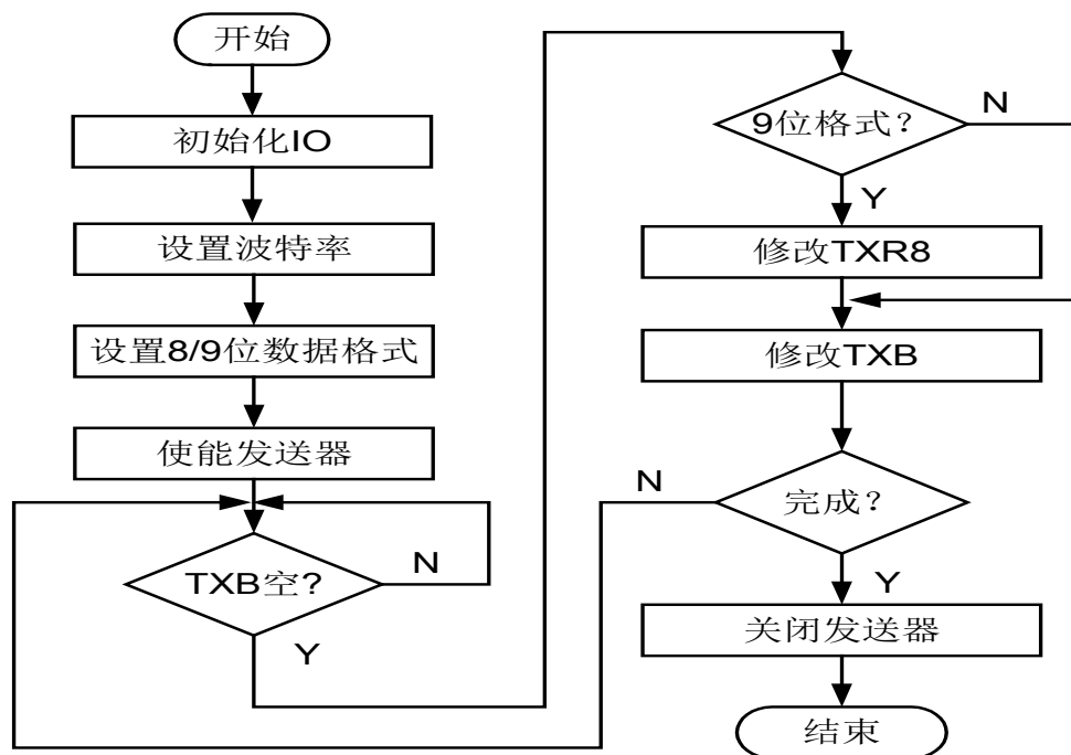
图 5-15 UART 发送器操作流程图
