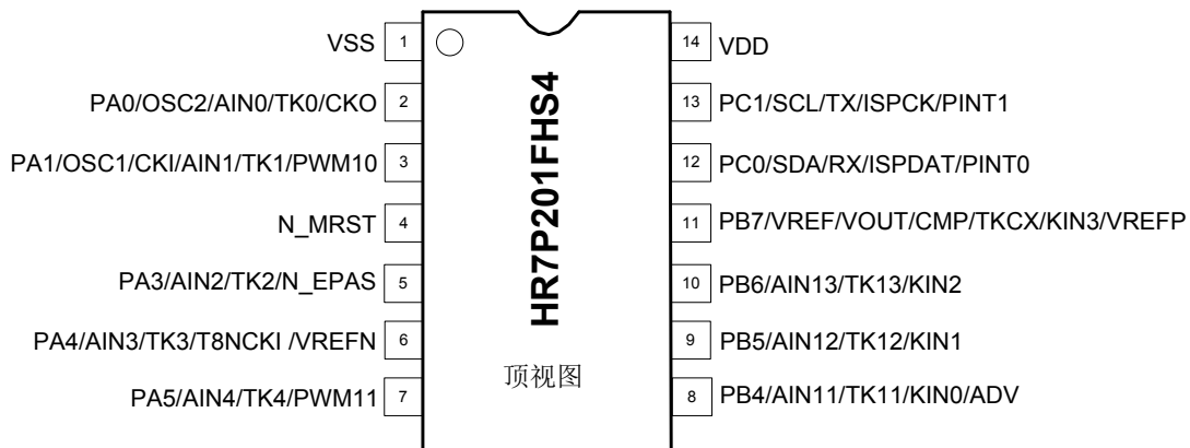
图 1-4 HR7P201（SOP14）顶视图
