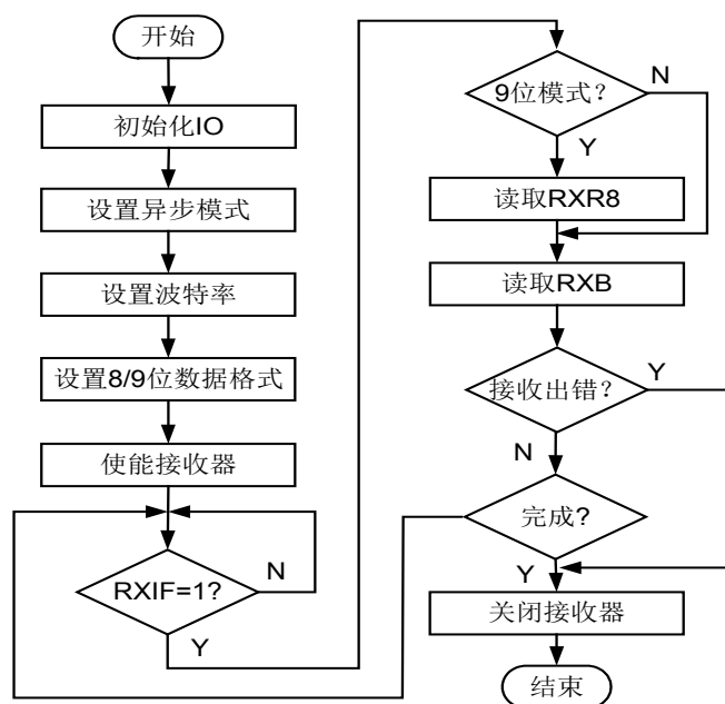
图 5-16 UART 接收器操作流程图
